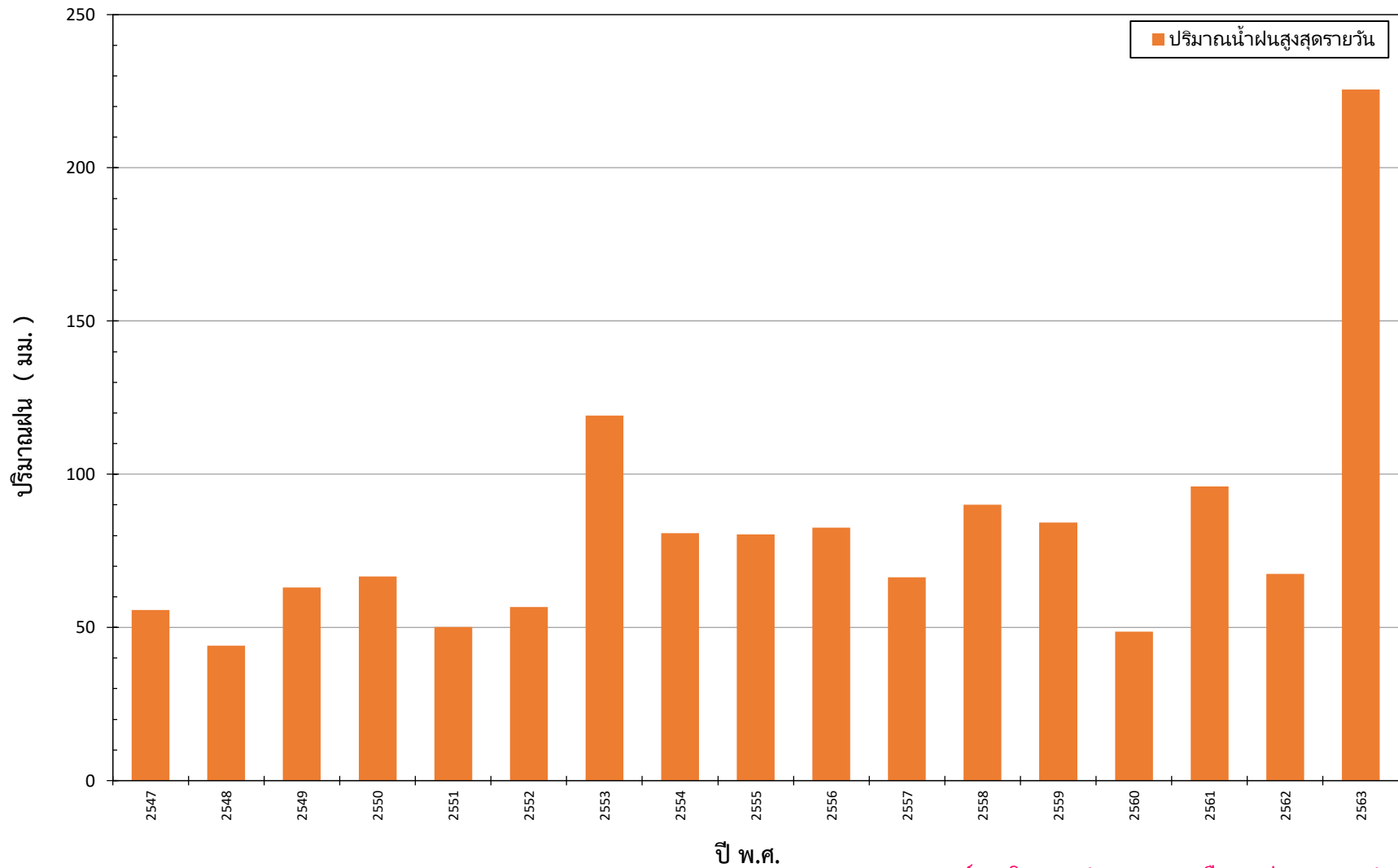
กราฟแสดงปริมาณฝนสูงสุดรายวัน ปีพ.ศ. 2547 - 2563 สถานีน้ำฝน S.42 ( 360790 ) อ.วิเชียรบุรี จ.เพชรบูรณ์
